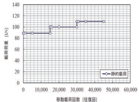
図-5 荷重と載荷回数の関係
